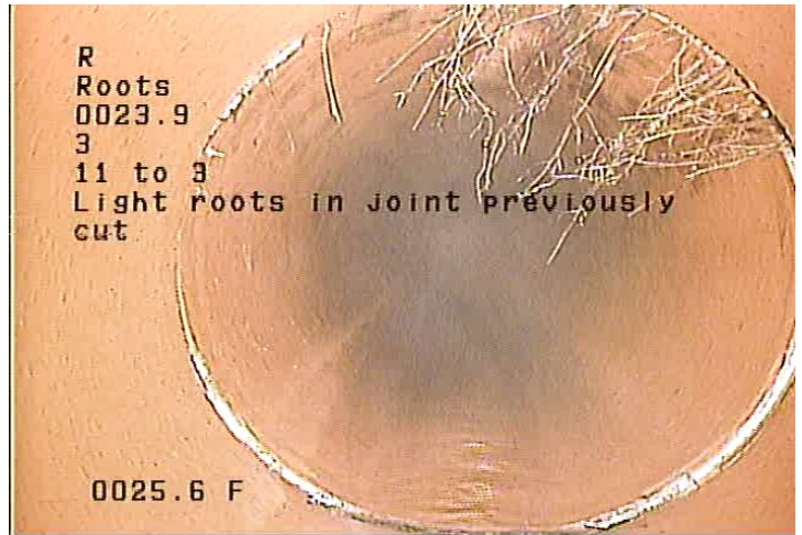
MH - Manhole @ 42.6 ft. End Manhole 40M08
